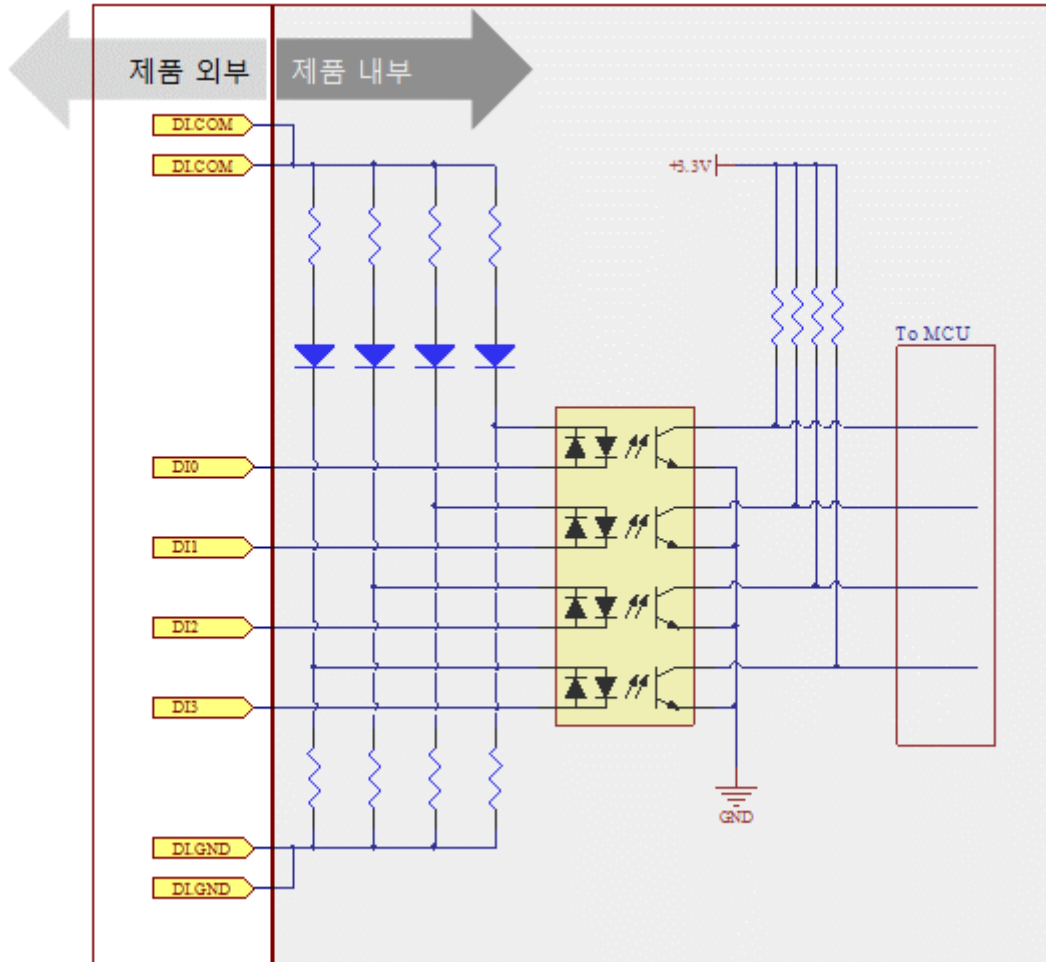
그림 1-5 디지털 입력 부 회로도
