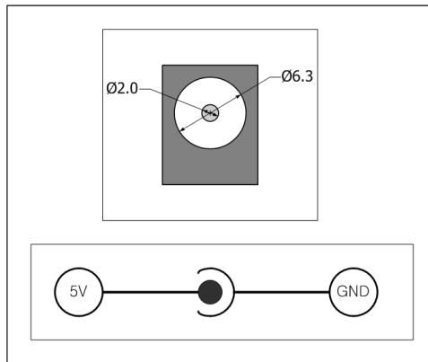
그림 1-3 PWR2 포트 사양
