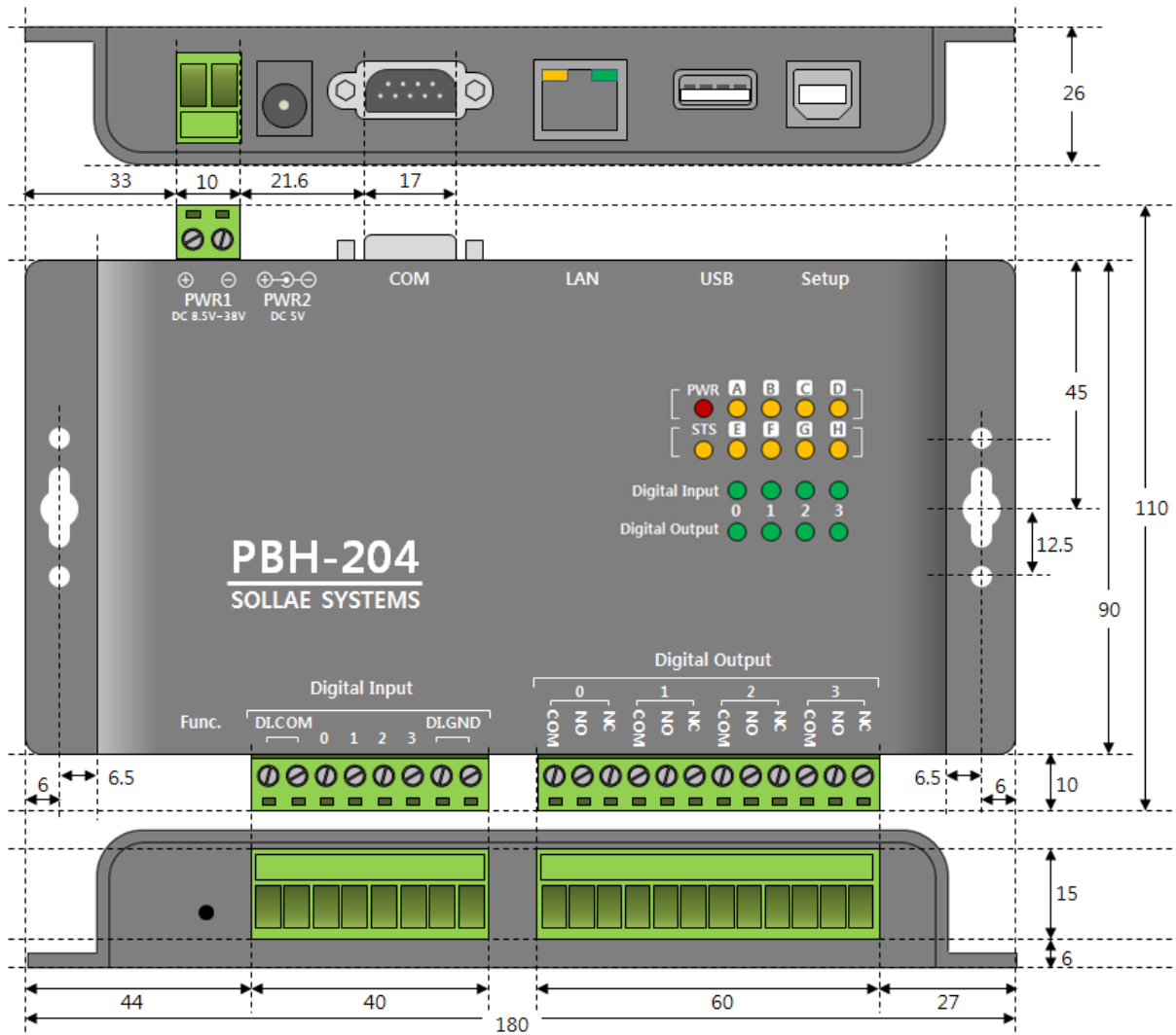
그림 1-1 치수
