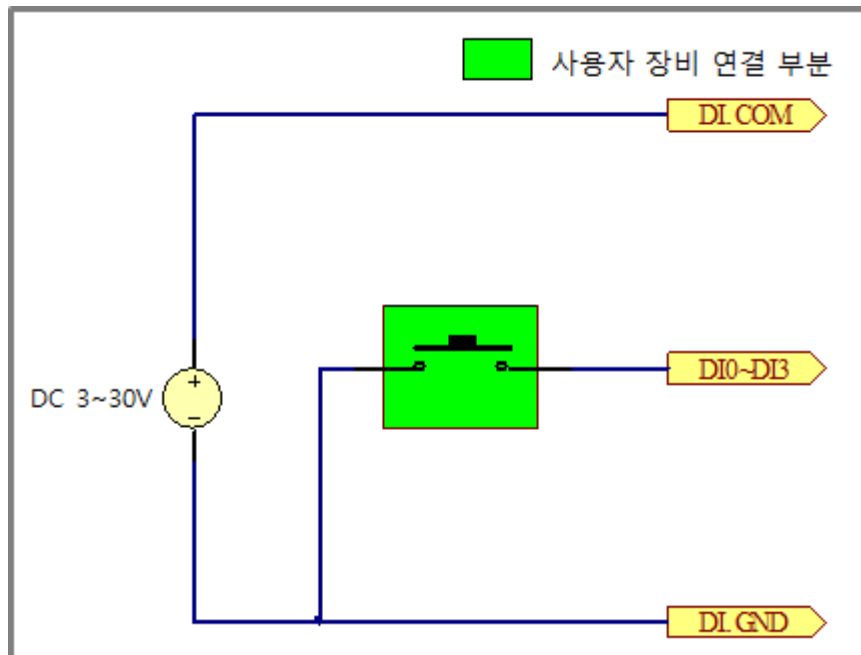
그림 1-7 접점 입력을 위한 사용자 장비 연결
