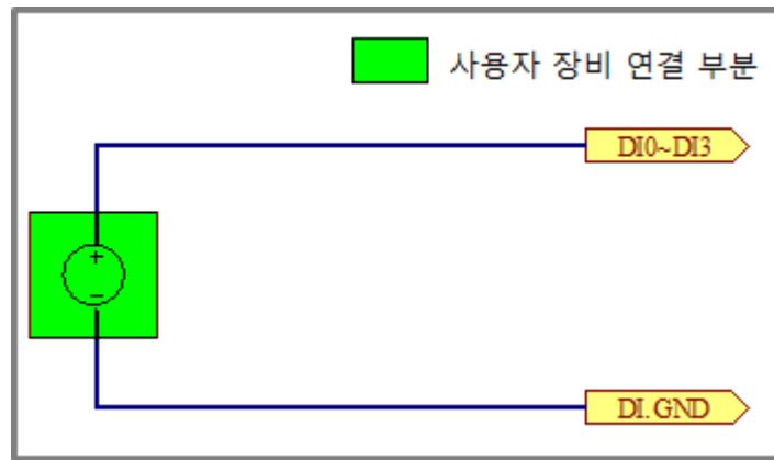
그림 1-6 전압 입력을 위한 사용자 장비 연결
