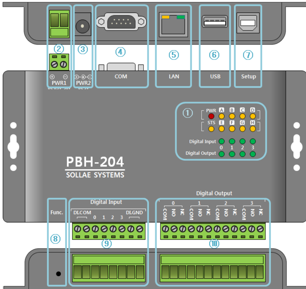
그림 1-2 패널 레이아웃
